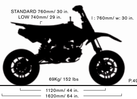
SM 125
